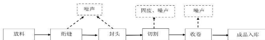
图 4.5-1 生产工艺及产污环节图
