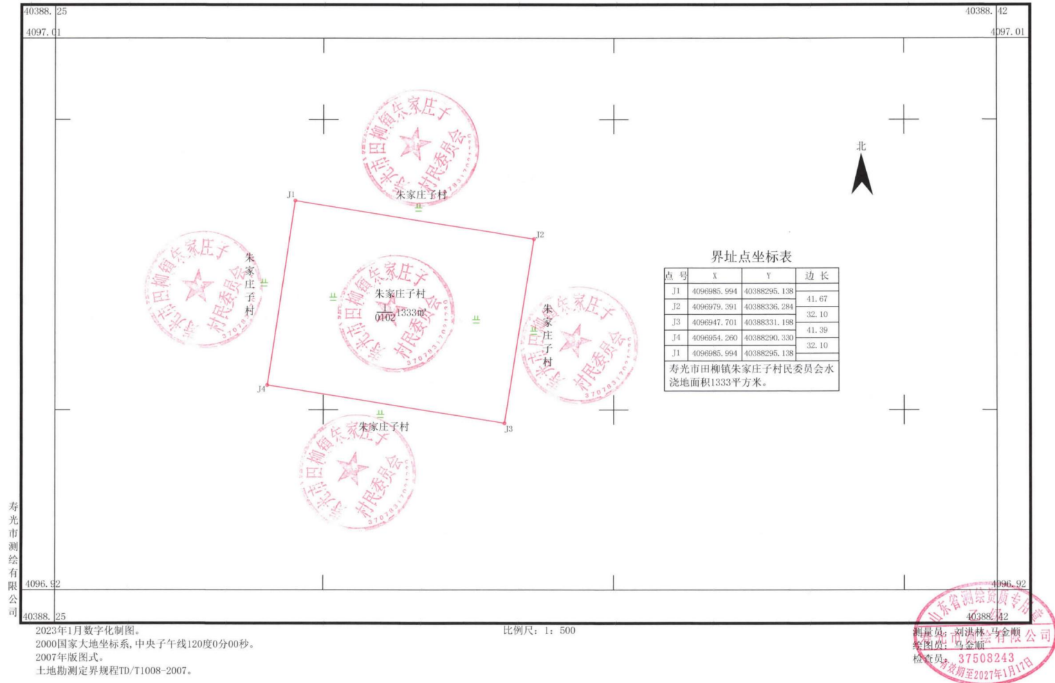
图 2.2-2 地块勘测定界图
