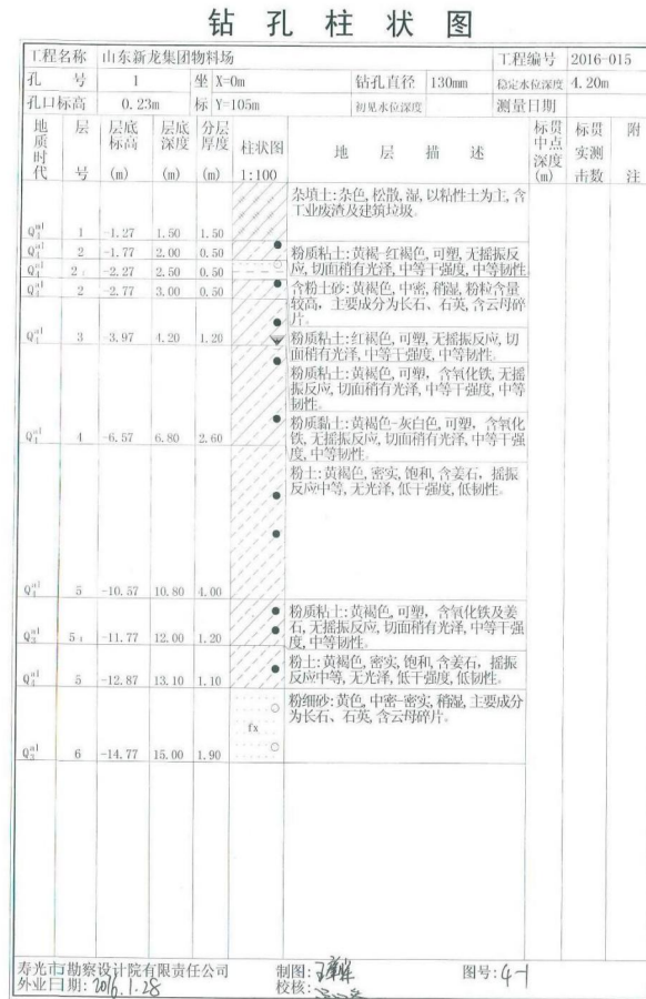
图 3.1-8 钻孔柱状图
