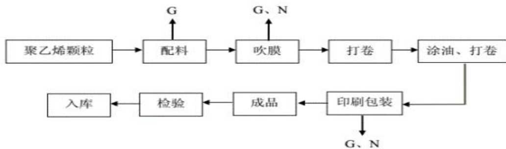
图 4.5-3 生产工艺及产污环节图 (G-废气, N-噪声)
