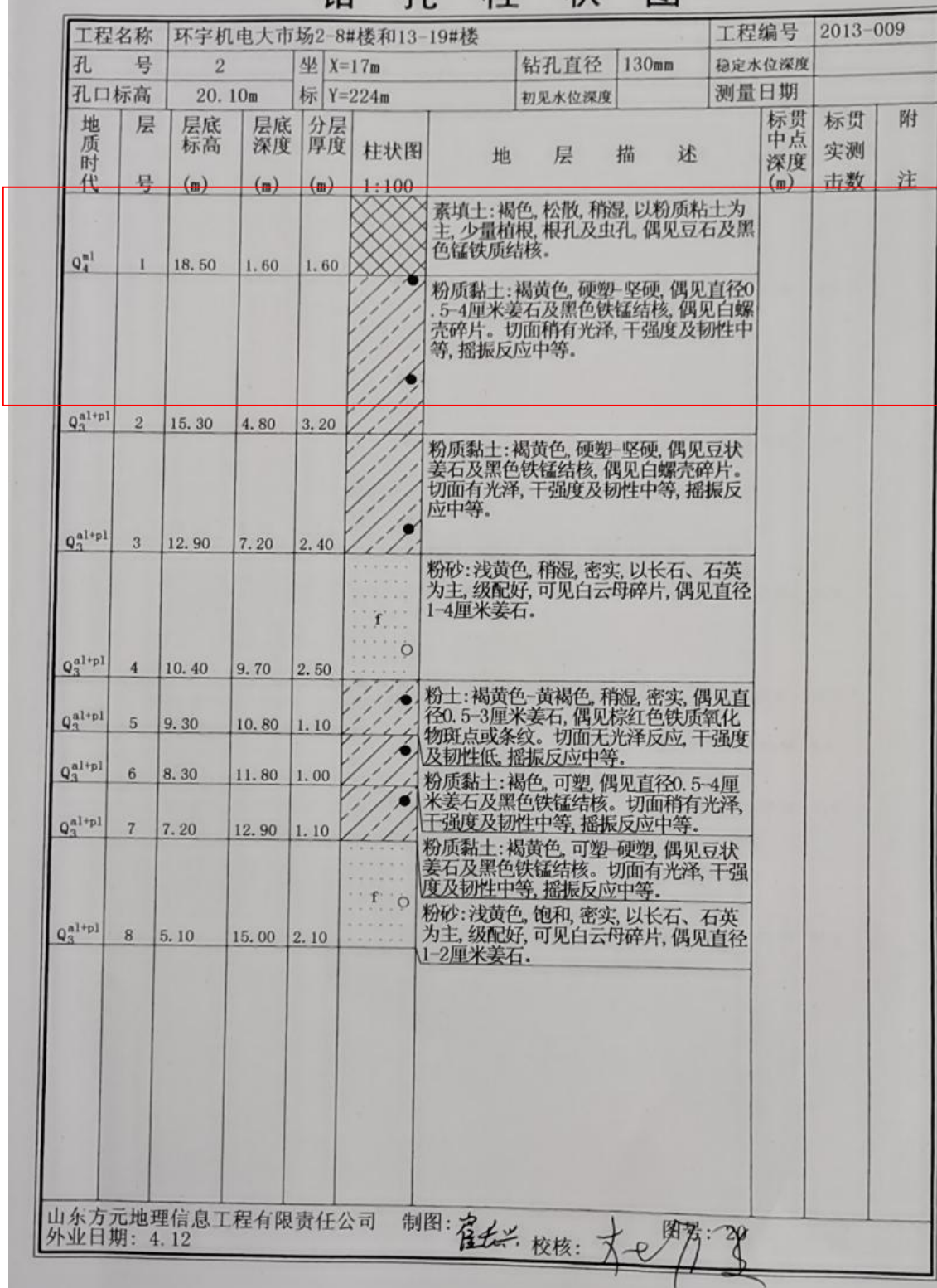
图 2.2-3 钻孔柱状图
